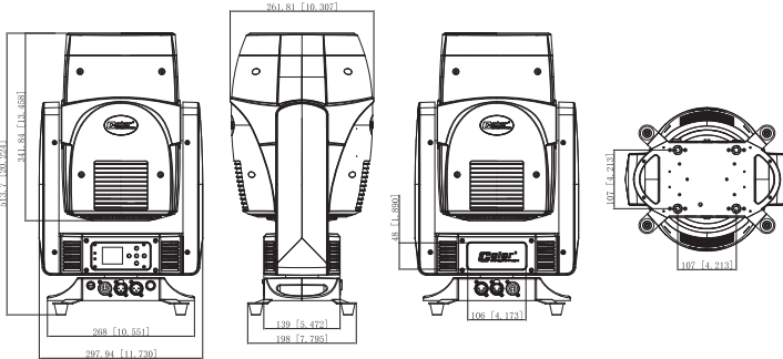
尺寸图
