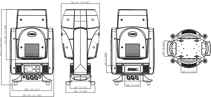
尺寸图
